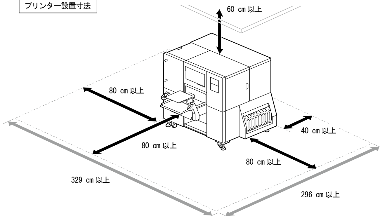
プリンター設置寸法
