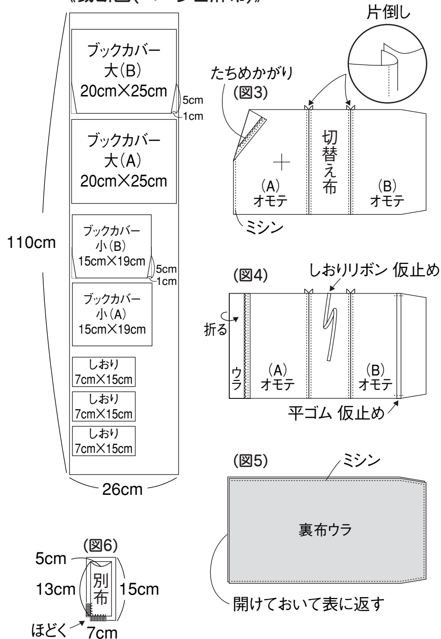
《裁断図(ベージュ麻布)》
